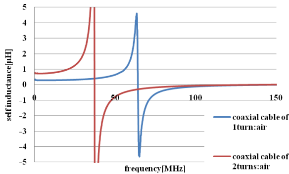
Fig.14 Self inductance without water as a function of frequency Fig.14 より、1 回巻コイルの等価回路を L_1 、 C_1 の並列回路とすると、
